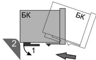
Рис. 3 Установка на “высокую” панель
